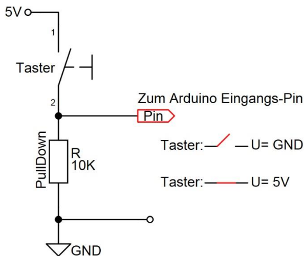
Abb. 9 Ein offener Eingang mit Pulldown-Widerstand
